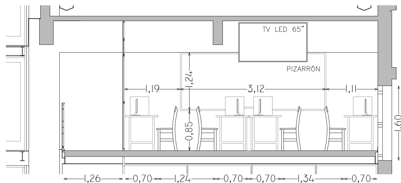
CORTE A-A
