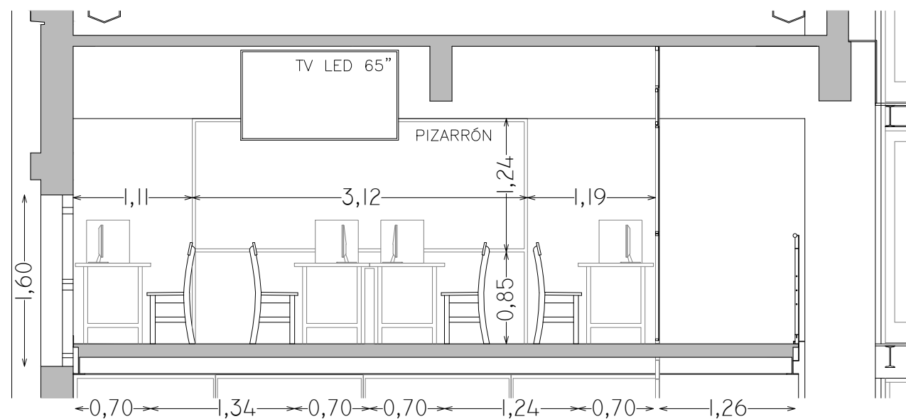
CORTE A-A
