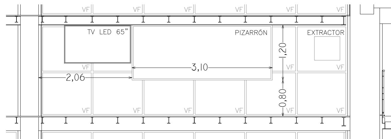
CORTE A-A
