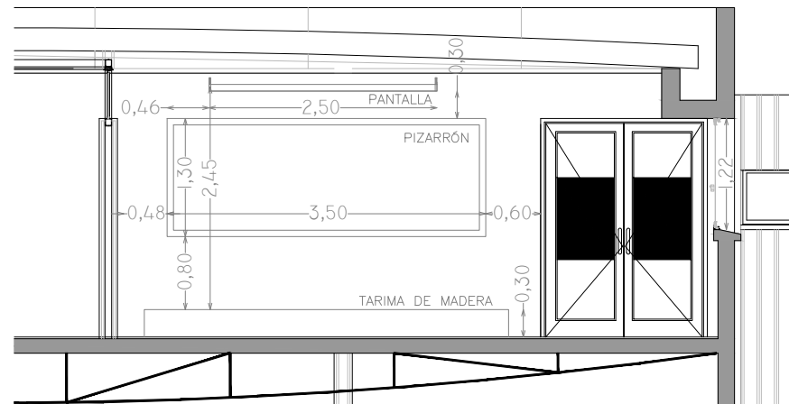
CORTE A-A
