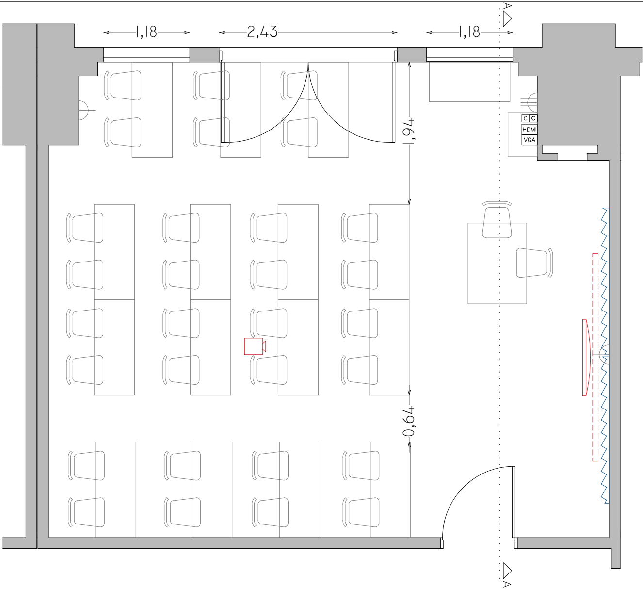
PLANTA
