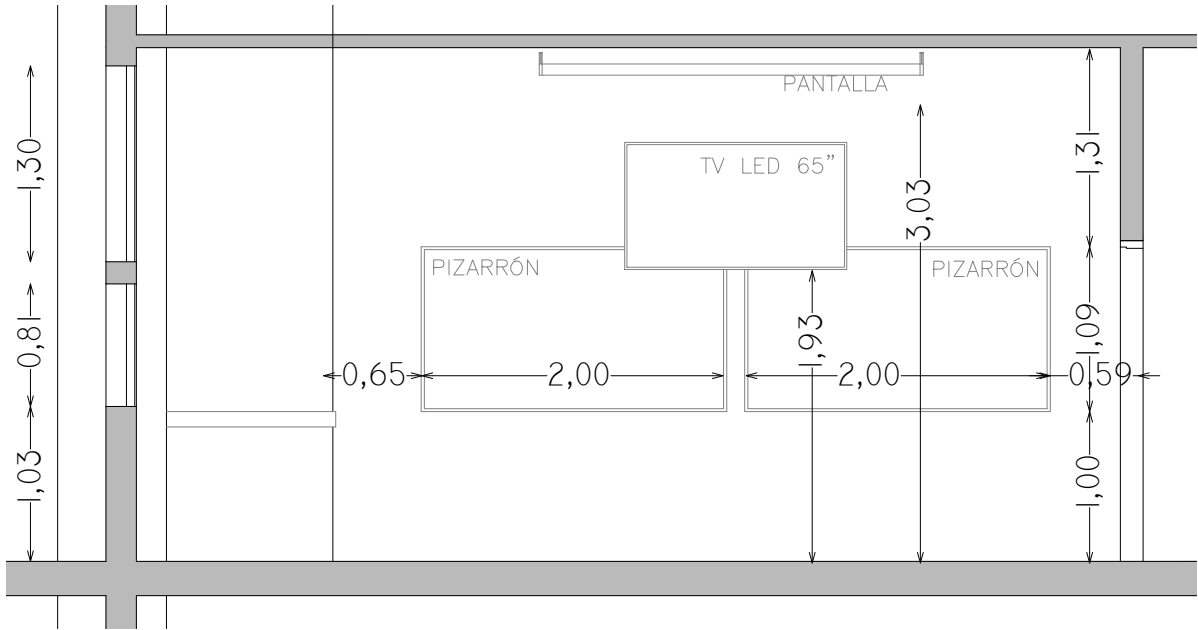
CORTE A-A
