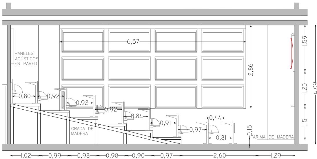
CORTE B-B
