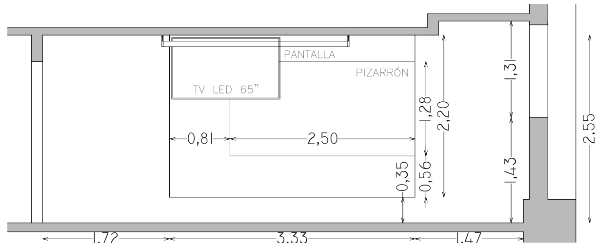
CORTE A-A
